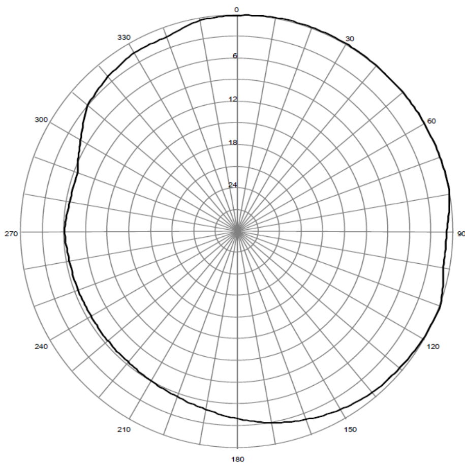
Pozioma charakterystyka promieniowania anteny stacji Kraków 96,70 MHz
