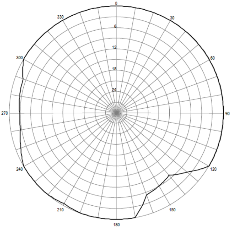
Pozioma charakterystyka promieniowania anteny stacji Elk 102,60 MHz
