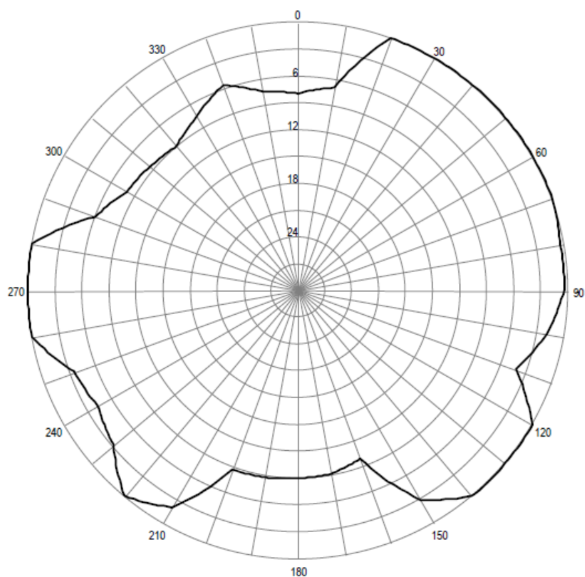
Pozioma charakterystyka promieniowania anteny stacji Stalowa Wola 93,50 MHz
