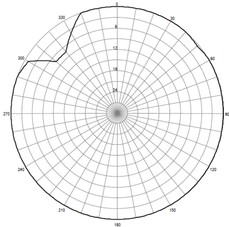
Pozioma charakterystyka promieniowania anteny stacji Krynica Góra Parkowa 104,60 MHz
