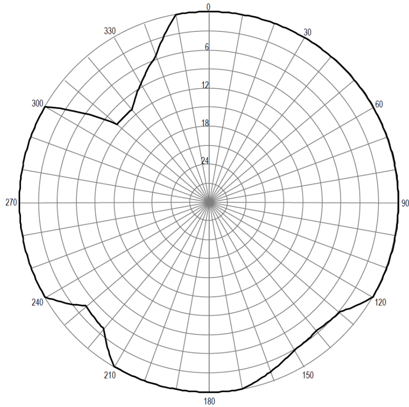
Pozioma charakterystyka promieniowania anteny stacji Iława 89,0 MHz
