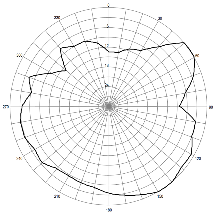
Pozioma charakterystyka promieniowania anteny stacji Jakubów 102,60 MHz
