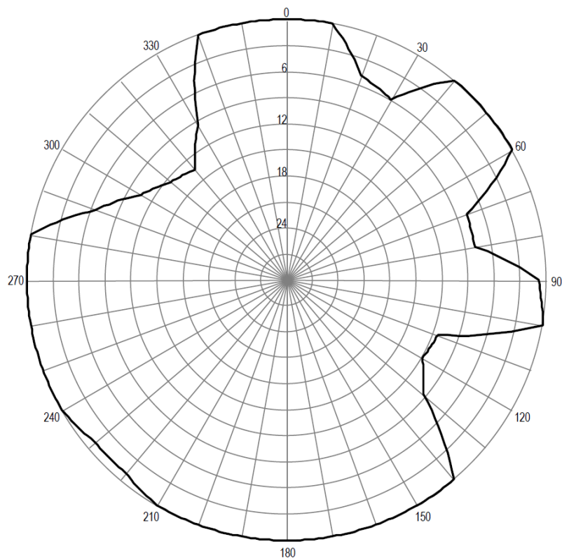
Pozioma charakterystyka promieniowania anteny stacji Zaniemyśl 95,20 MHz
