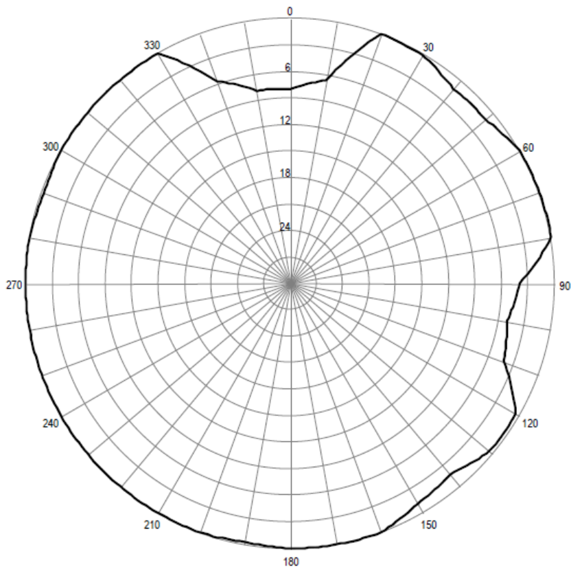
Pozioma charakterystyka promieniowania anteny stacji Radom 106,20 MHz
