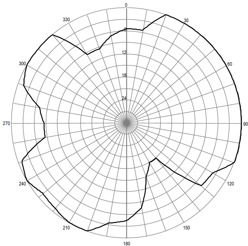
Pozioma charakterystyka promieniowania anteny stacji Efk 90,10 MHz
