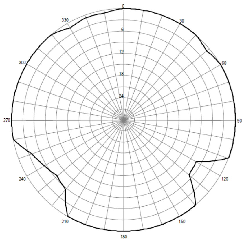
Pozioma charakterystyka promieniowania anteny stacji Poznań 104,70 MHz
