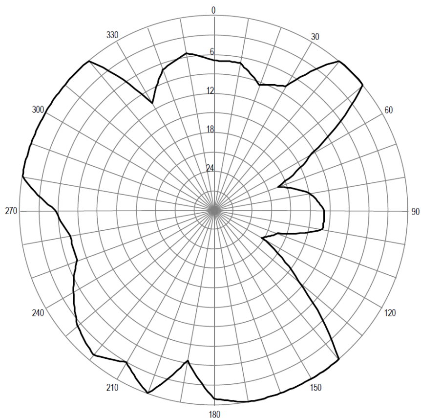
Pozioma charakterystyka promieniowania anteny stacji Dobromierz 94,40 MHz
