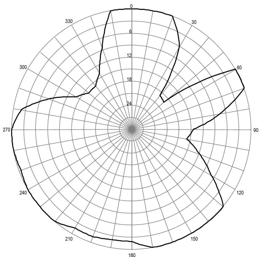
Pozioma charakterystyka promieniowania anteny stacji Kielce Św. Krzyż 91,30 MHz
