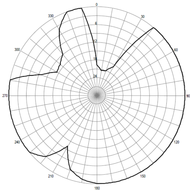
Pozioma charakterystyka promieniowania anteny stacji Płock 88,10 MHz
