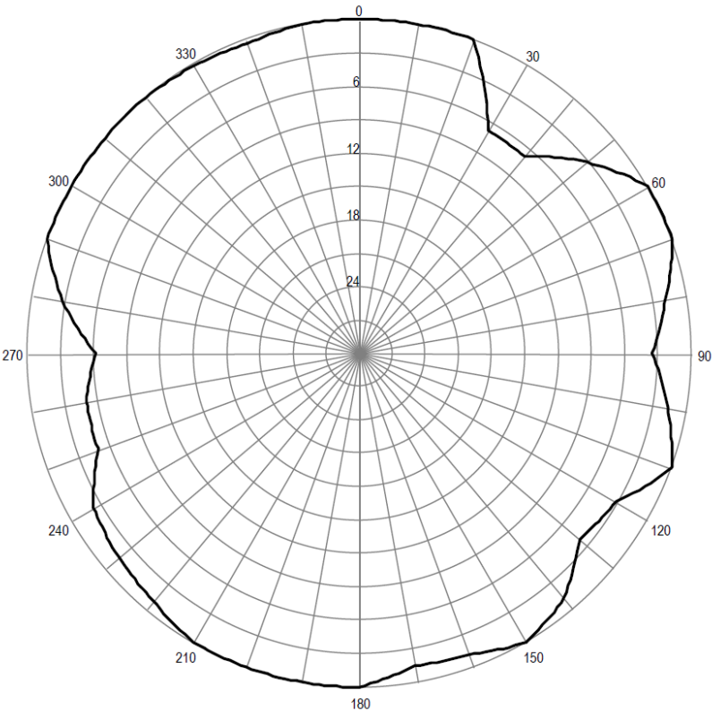
Pozioma charakterystyka promieniowania anteny stacji Jakubów 103,80 MHz
