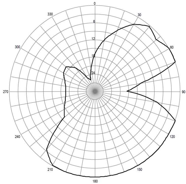
Pozioma charakterystyka promieniowania anteny stacji Jakubów 88,20 MHz
