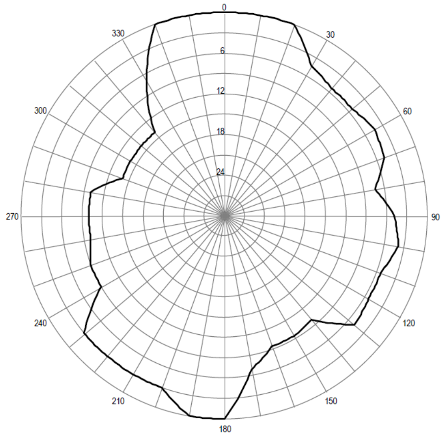
Pozioma charakterystyka promieniowania anteny stacji Szczecin 98,90 MHz
