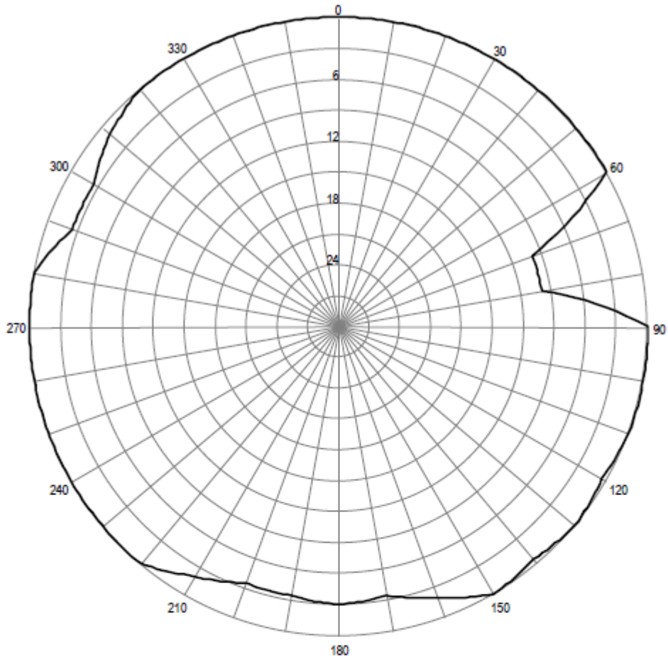
Pozioma charakterystyka promieniowania anteny stacji Bolesławiec 88,50 MHz
