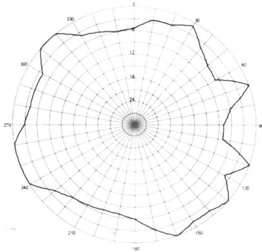
Pozioma charakterystyka promieniowania anteny stacji Września 93,70 MHz
