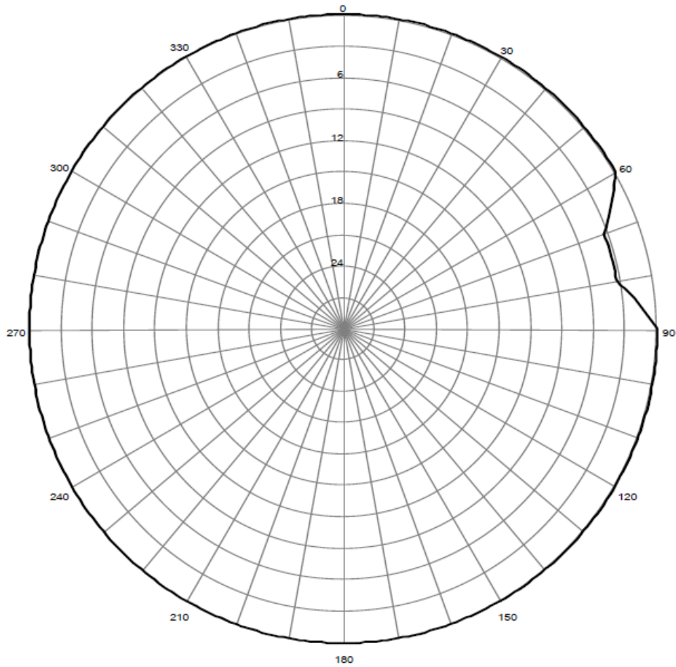
Pozioma charakterystyka promieniowania anteny stacji Strzegom 101,70 MHz
