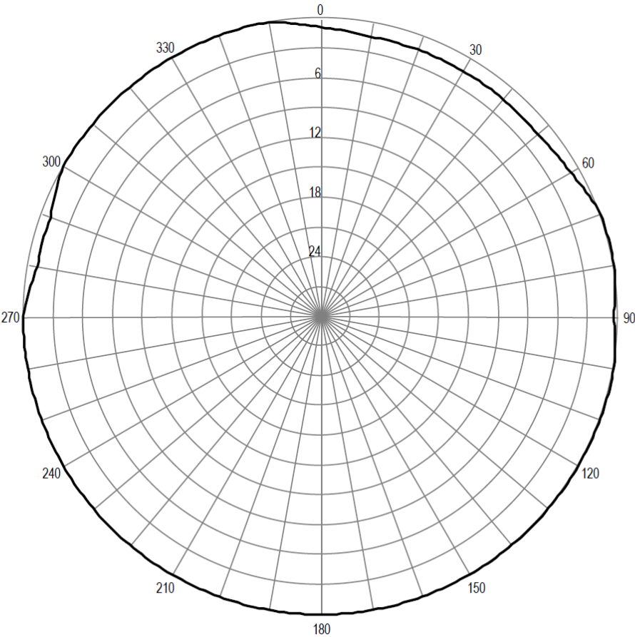
Pozioma charakterystyka promieniowania anteny stacji Toruń 104,60 MHz
