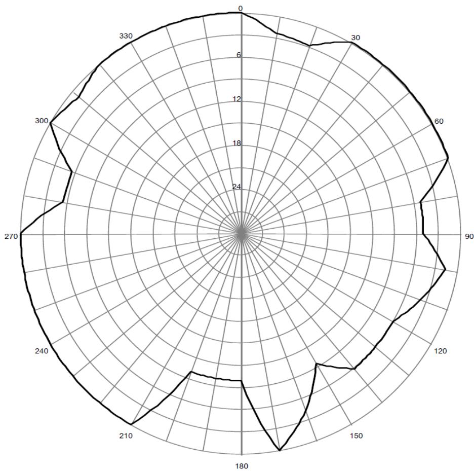
Pozioma charakterystyka promieniowania anteny stacji Limanowa G. Miejska 100,30 MHz
