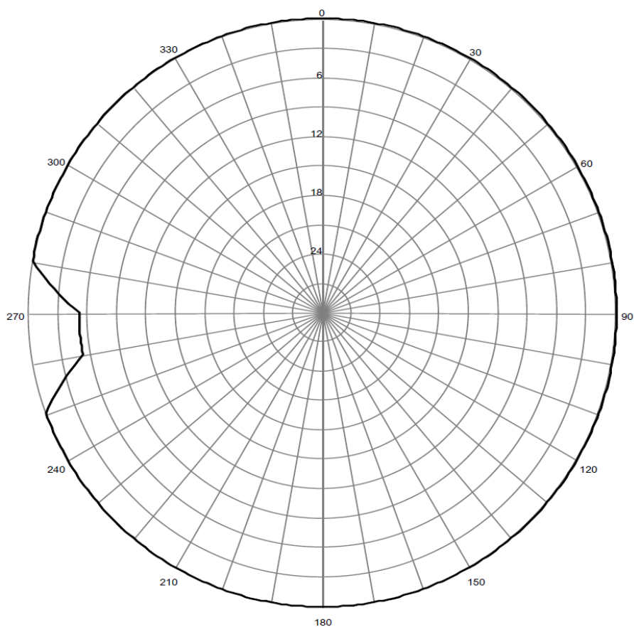
Pozioma charakterystyka promieniowania anteny stacji Sochaczew 94,90 MHz
