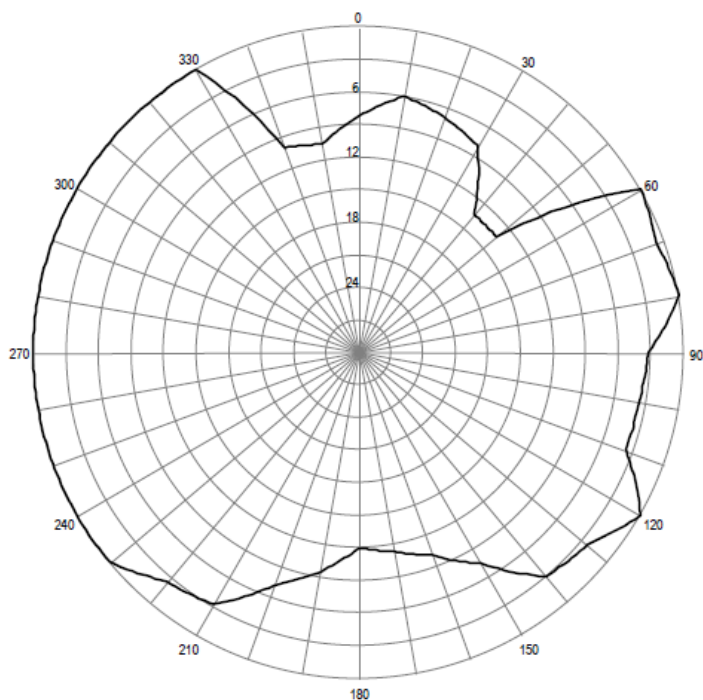
Pozioma charakterystyka promieniowania anteny stacji Starogard Gdański 89,80 MHz
