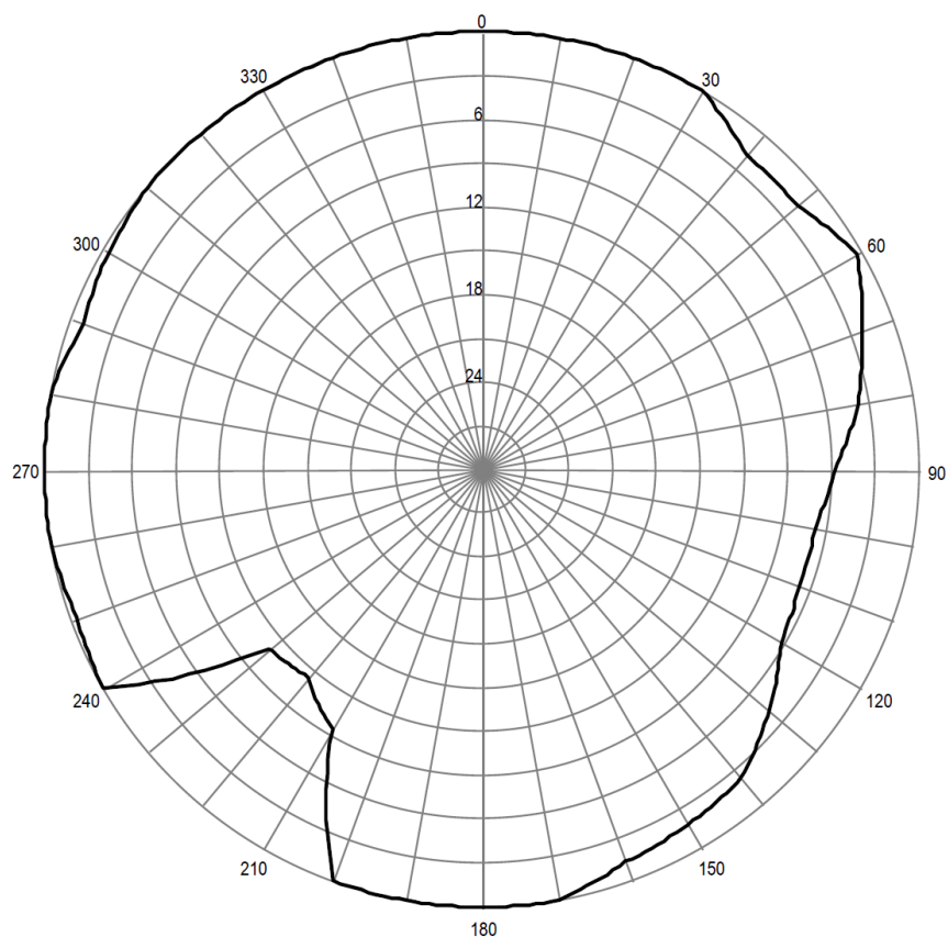
Pozioma charakterystyka promieniowania anteny stacji Tarnobrzeg 99,10 MHz
