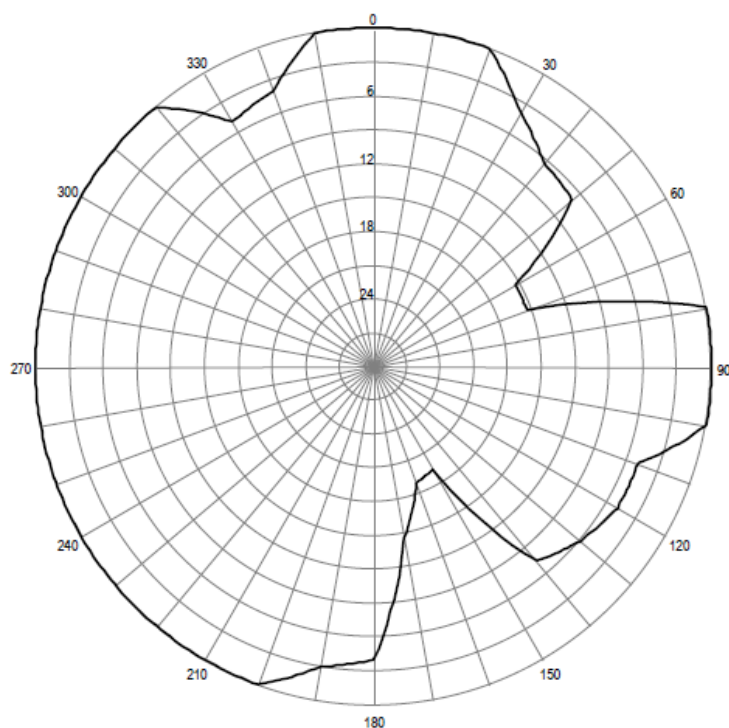
Pozioma charakterystyka promieniowania anteny stacji Świdnica 101,70 MHz
