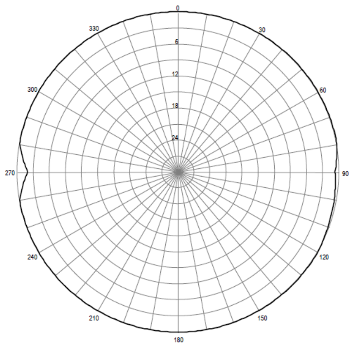
Pozioma charakterystyka promieniowania anteny stacji Słupsk 92,10 MHz
