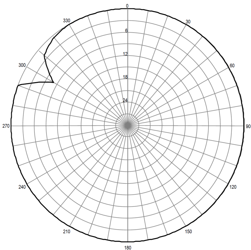
Pozioma charakterystyka promieniowania anteny stacji Goleniów 101,0 MHz
