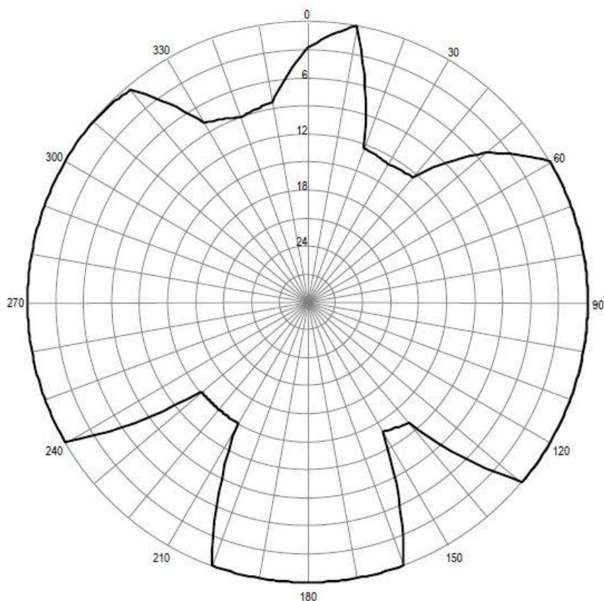
Pozioma charakterystyka promieniowania anteny stacji Wola k/ Czerwińska 99,90 MHz
