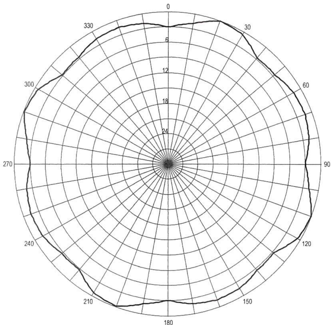
Pozioma charakterystyka promieniowania anteny stacji WARSZAWA PKiN 95,80 MHz
