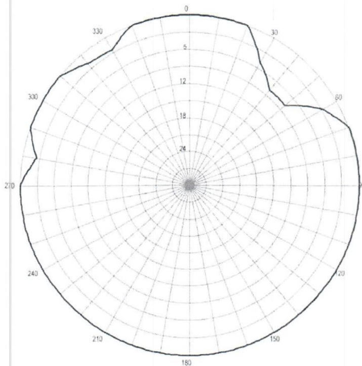
Pozioma charakterystyka promieniowania anteny stacji Oświęcim 94,9 MHz
