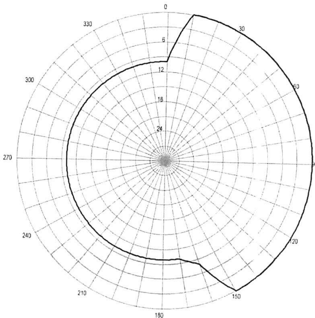
Pozioma charakterystyka promieniowania anteny stacji Jerzykowice Wielkie 88,7 MHz
