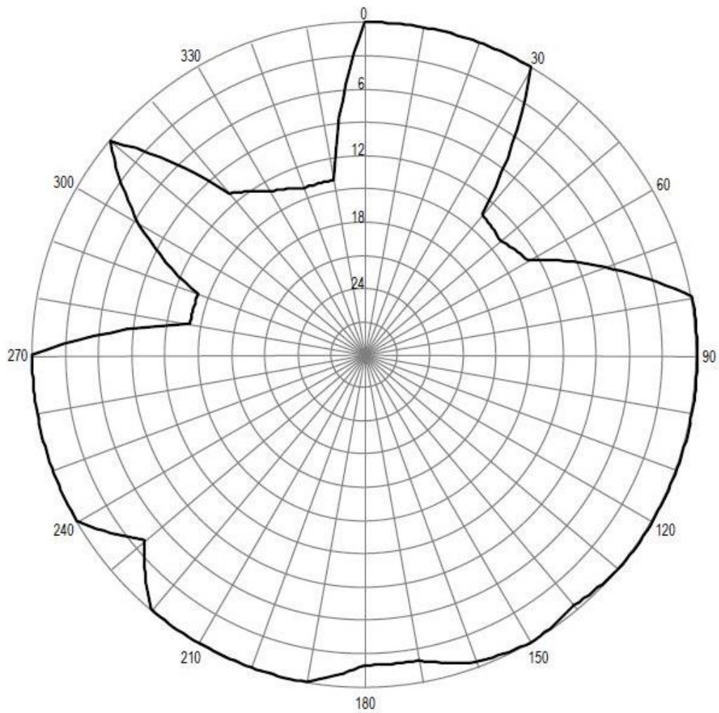
Pozioma charakterystyka promieniowania anteny stacji Tarnowskie Góry 100,0 MHz
