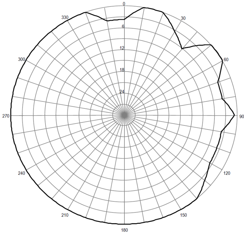
Pozioma charakterystyka promieniowania anteny stacji Szpetal Górny 100,90 MHz
