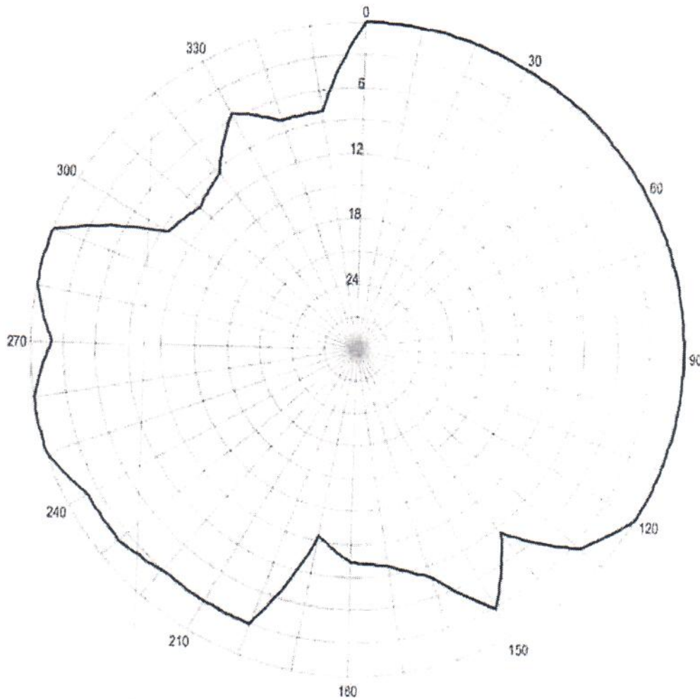
Pozioma charakterystyka promieniowania anteny stacji Wierzbicice 103,60 MHz
