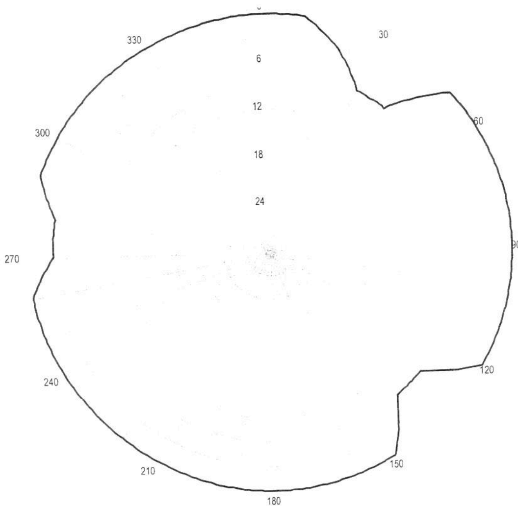
Pozioma charakterystyka promieniowania anteny stacji
