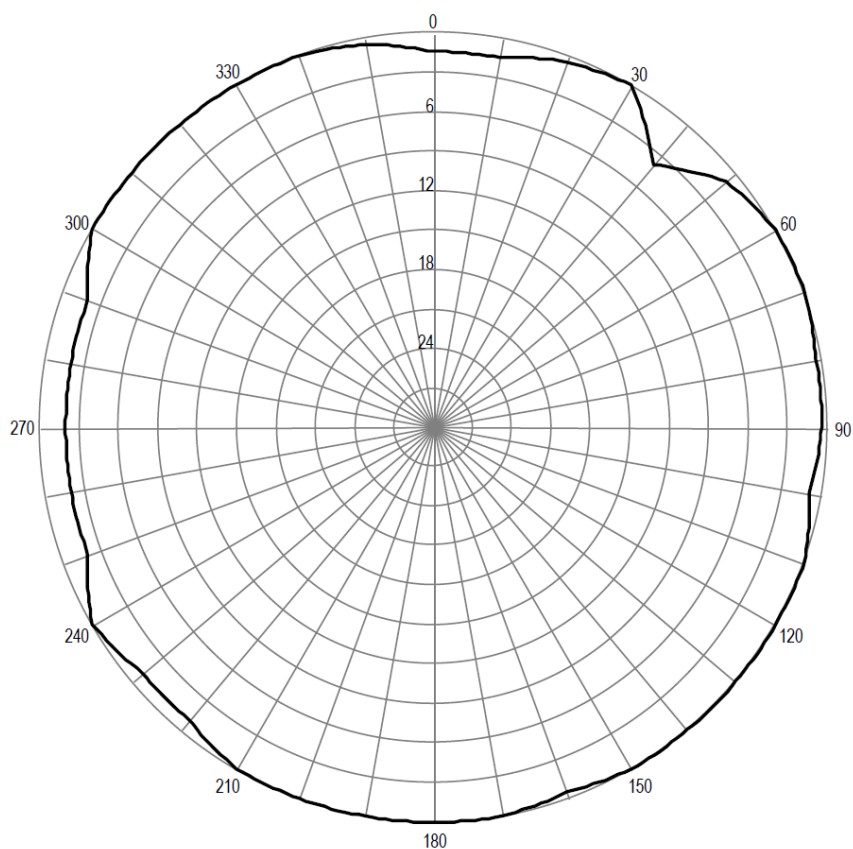
Pozioma charakterystyka promieniowania anteny stacji Toruń 88,80 MHz
