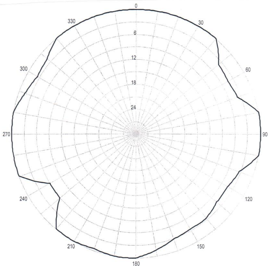
Pozioma charakterystyka promieniowania anteny stacji Zielona Góra 89,00 MHz
