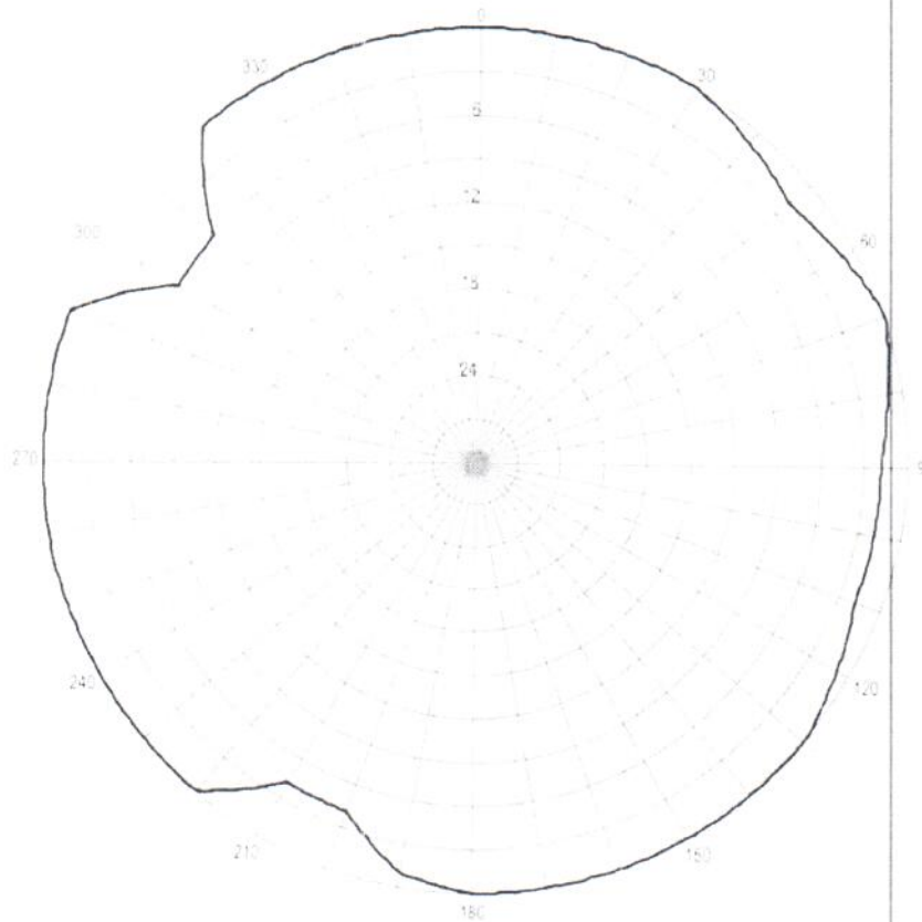
Pozioma charakterystyka promieniowania anteny stacji Sieradz 104,7 MHz
