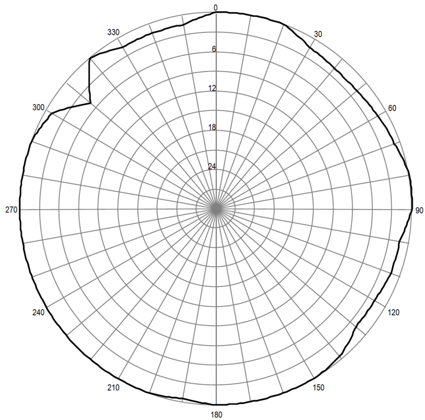
Pozioma charakterystyka promieniowania anteny stacji Toruń 92,80 MHz
