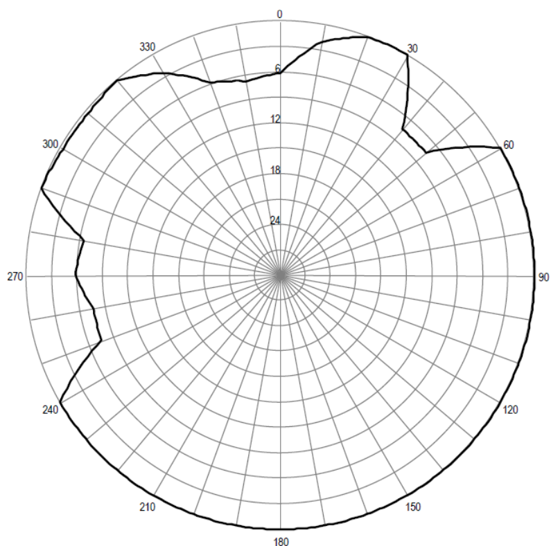
Pozioma charakterystyka promieniowania anteny stacji Bochnia 97,00 MHz
