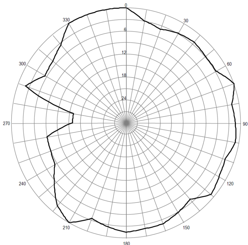
Pozioma charakterystyka promieniowania anteny stacji Poznań Mosina 97,00 MHz
