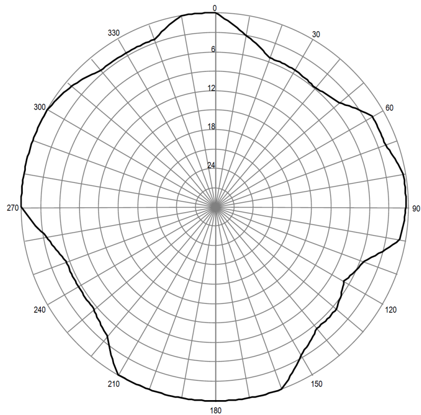
Pozioma charakterystyka promieniowania anteny stacji Wrocław 92,0 MHz
