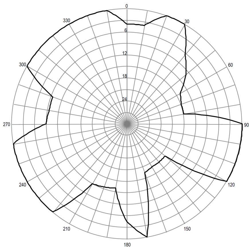
Pozioma charakterystyka promieniowania anteny stacji Ciechanów 88,70 MHz
