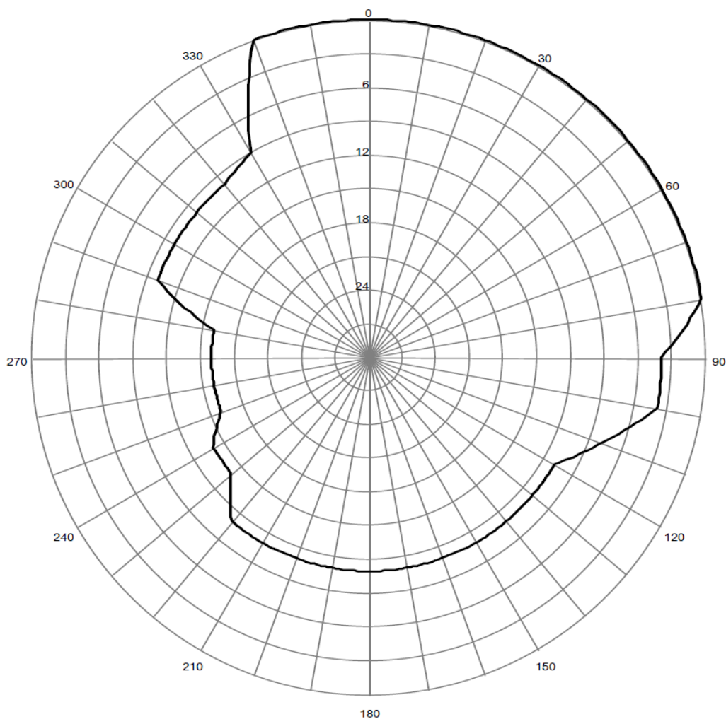
Pozioma charakterystyka promieniowania anteny stacji Wałbrzych G. Chelmiec 90,90 MHz
