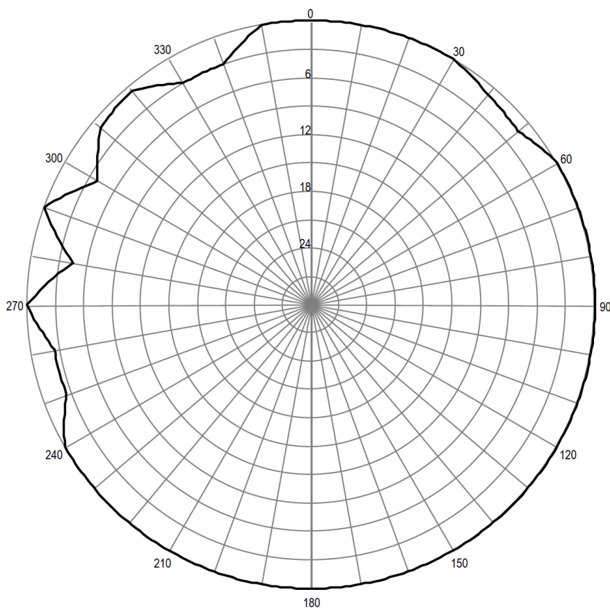
Pozioma charakterystyka promieniowania anteny stacji Zakopane 105,20 MHz
