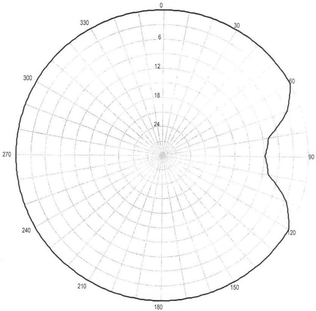
Pozioma charakterystyka promieniowania anteny stacji Radom 94,2 MHz
