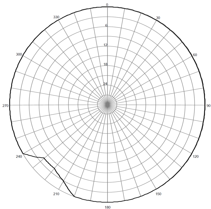
Pozioma charakterystyka promieniowania anteny stacji Regnów 94,70 MHz
