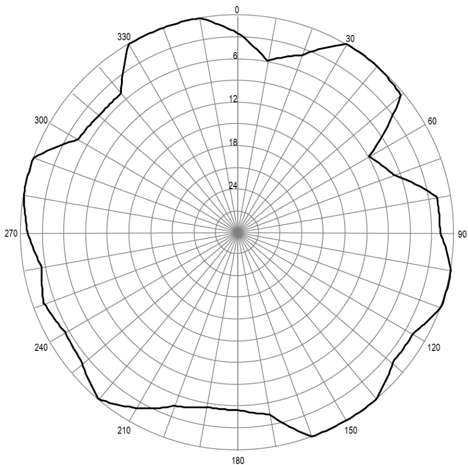
Pozioma charakterystyka promieniowania anteny stacji Gajewo k/ Giżycka 93,50 MHz
