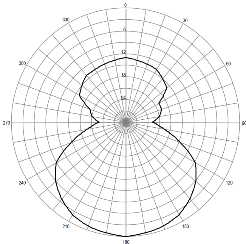
Pozioma charakterystyka promieniowania anteny stacji Wejherowo 102,6 MHz
