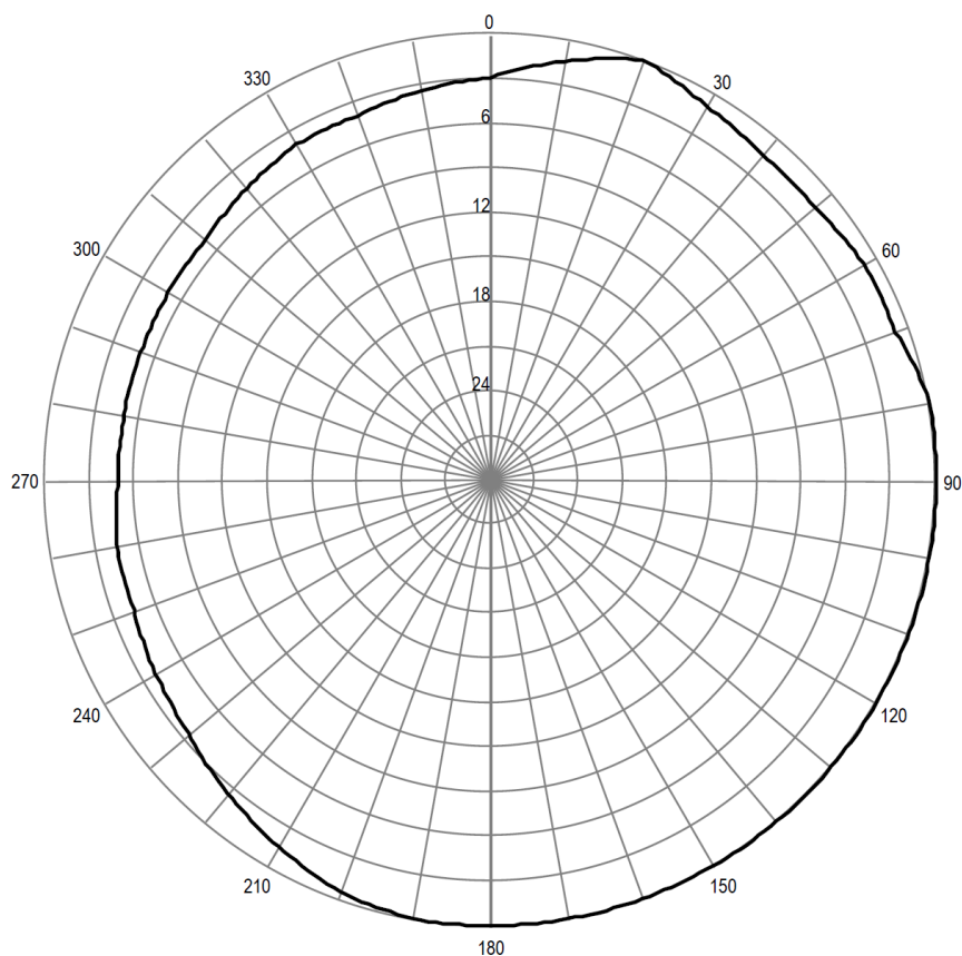
Pozioma charakterystyka promieniowania anteny stacji Warszawa 99,50 MHz
