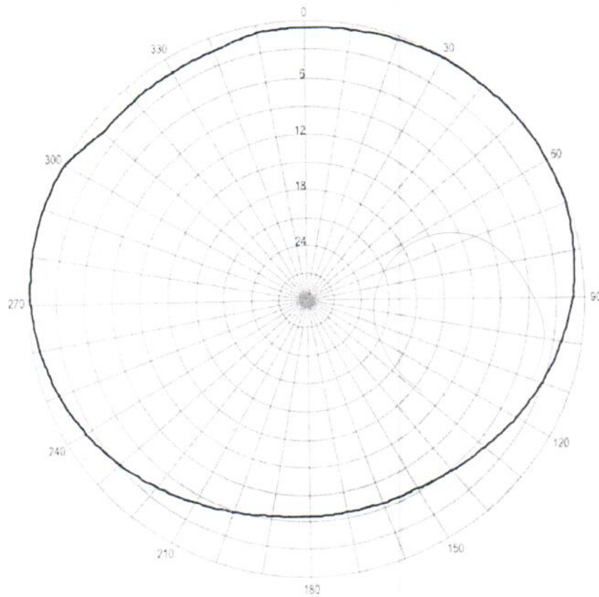
Pozioma charakterystyka promieniowania anteny stacji Góra Szyndzielnia 106,7 MHz
